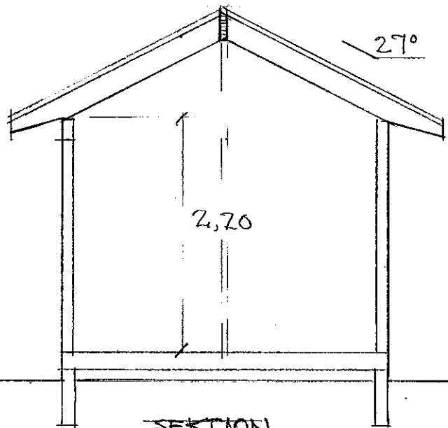
SEKTION
